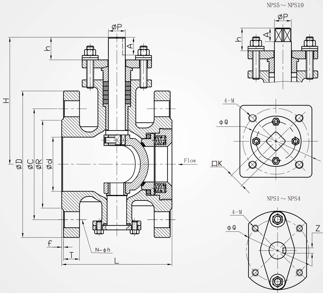
ASME Class300 DIMENSION TABLE
