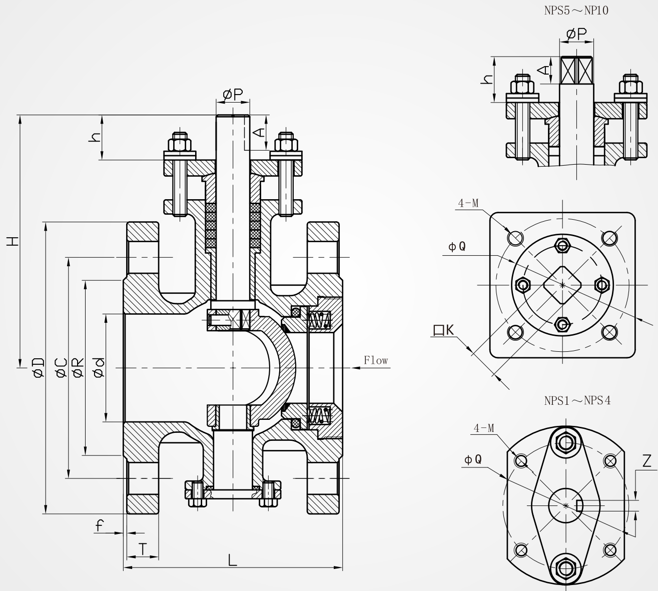
ASME Class150 DIMENSION TABLE
