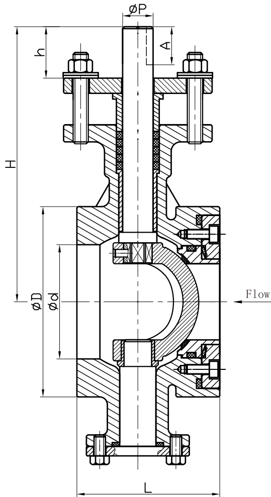
对夹式V型球阀尺寸图
